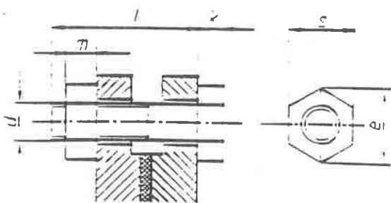
Abb. 1.4 Sechskantschraube mit Sechskantmutter in einer Flanschverbindung; vereinfachte Darstellung. l Schraubenlänge, d Gewindedurchmesser, k Kopfhöhe \approx 0.7 \cdot d , m Mutterhöhe \approx 0.8 \cdot d , e Eckenmaß \approx 2 \cdot d , s Schlüsselweite.
