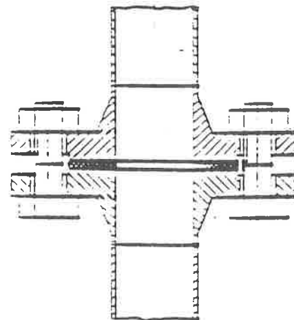
Abb. 1.3 Flanschverbindung, Vollschnitt.
