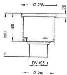
Ablaufkörper aus Kunststoff 67 050 | DN 125, Auslauf senkrecht
