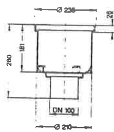
Ablaufkörper aus Kunststoff, DN 100 Auslauf senkrecht 67 040
