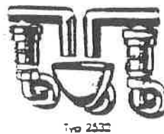
2 βαλβίδες εξαερισμού 1/2" με κοινή χωνί 1/2
