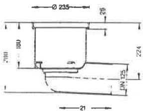
Ablaufkörper aus Kunststoff 67 010 | DN 125, Auslauf seitlich 2.5°
