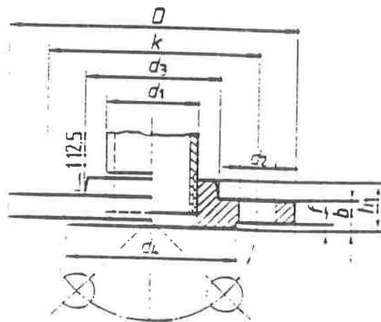
Abb. 1.5 Gewindeflansch nach DIN 2566. Haltschnrht.
