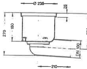
Ablaufkörper aus Kunststoff, DN 100 Auslauf seitlich 2.5° 67 000
